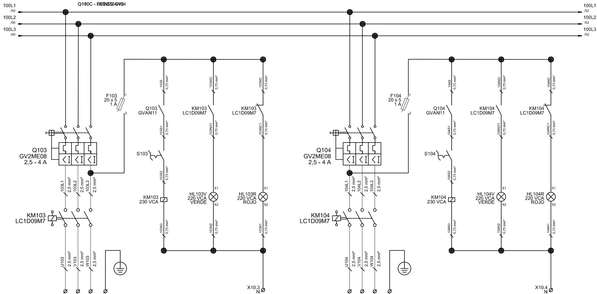
EXTRACTOR DE AIRE 2 EVAPORADOR
