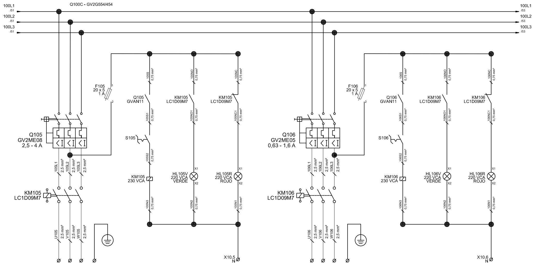
EXTRACTOR DE AIRE 2 CALENTADOR
